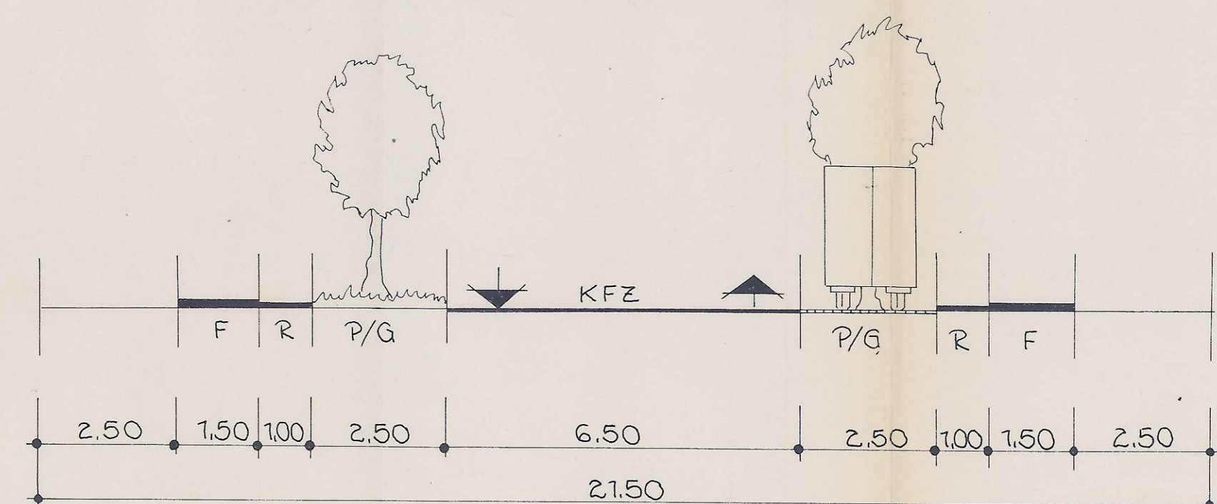
Straßenprofil (Maßstab 1:100)
