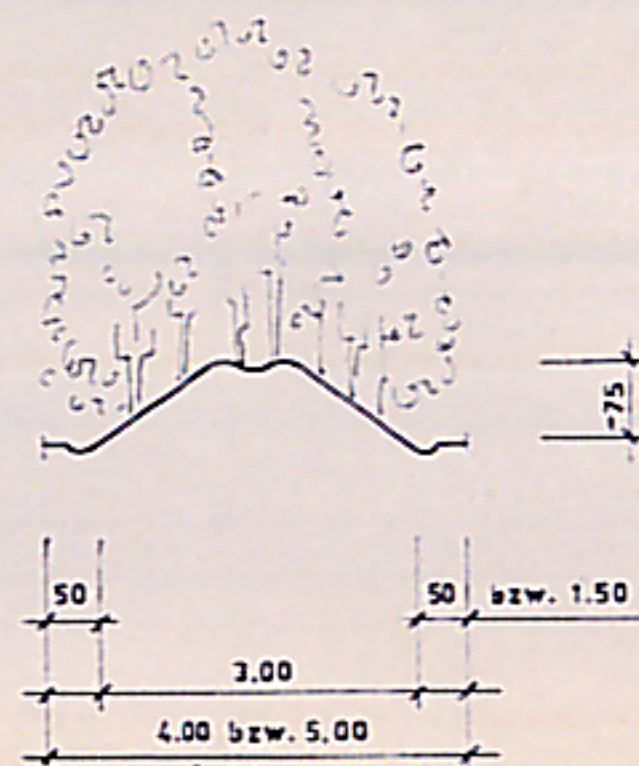
Knickwallprofil B - B, M 1:100
