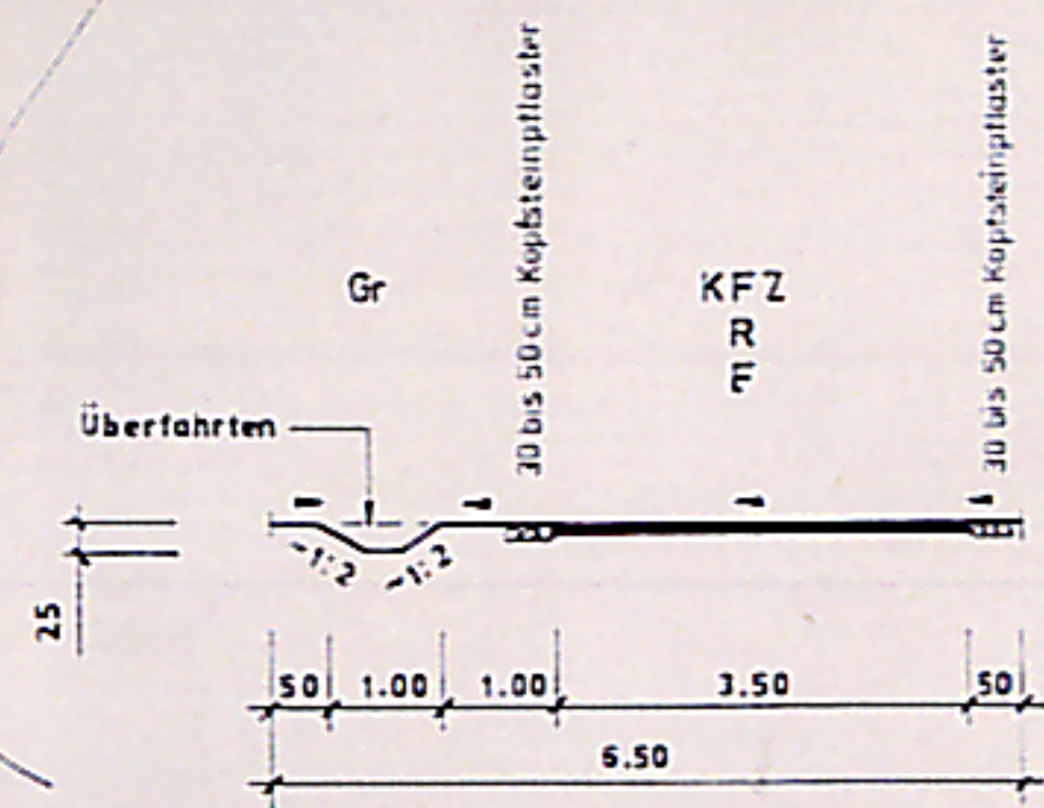
Straßenprofil A - A, M 1:100
