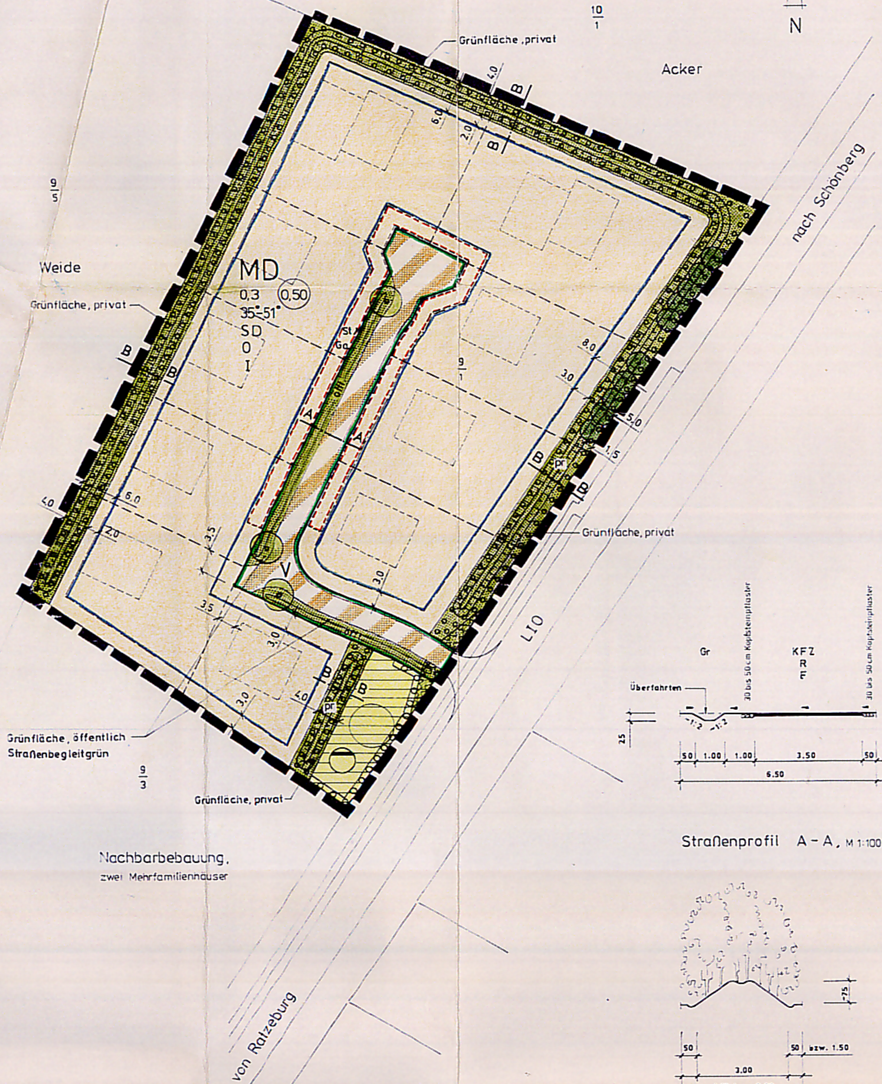
Knickwallprofil B - B, M 1:100
