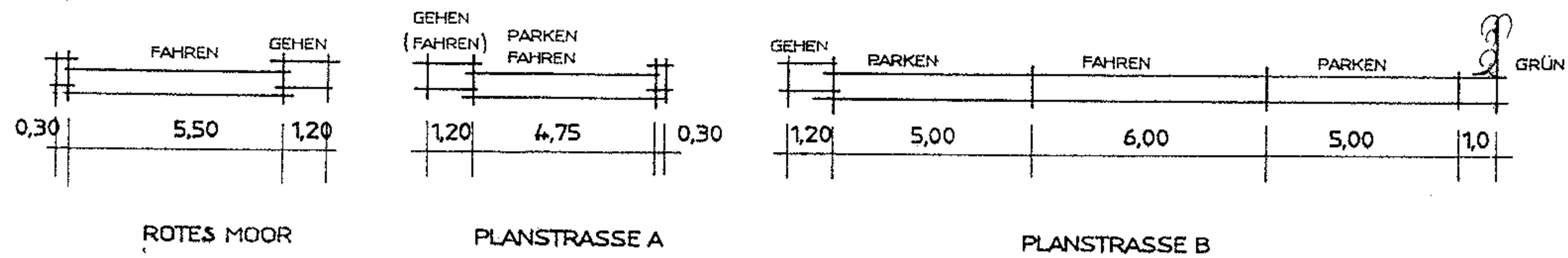
STRASSENQUERSCHNITTE
